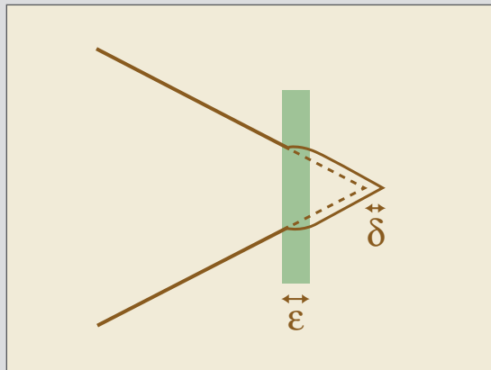
Ein Filter zwischen Teleskop und Kamera verschiebt die Fokusebene nach hinten.
